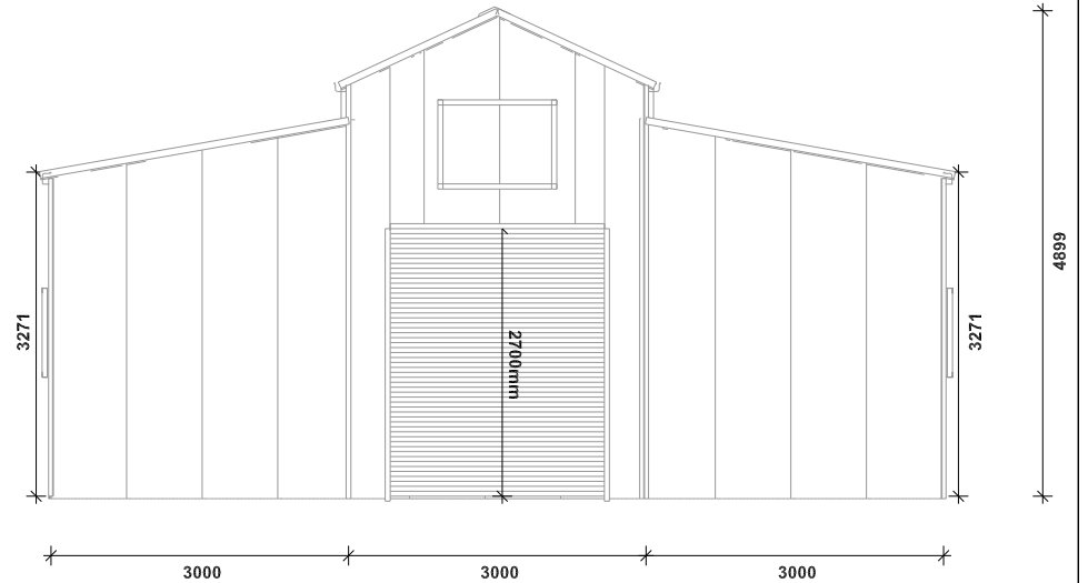
Elevation 4
