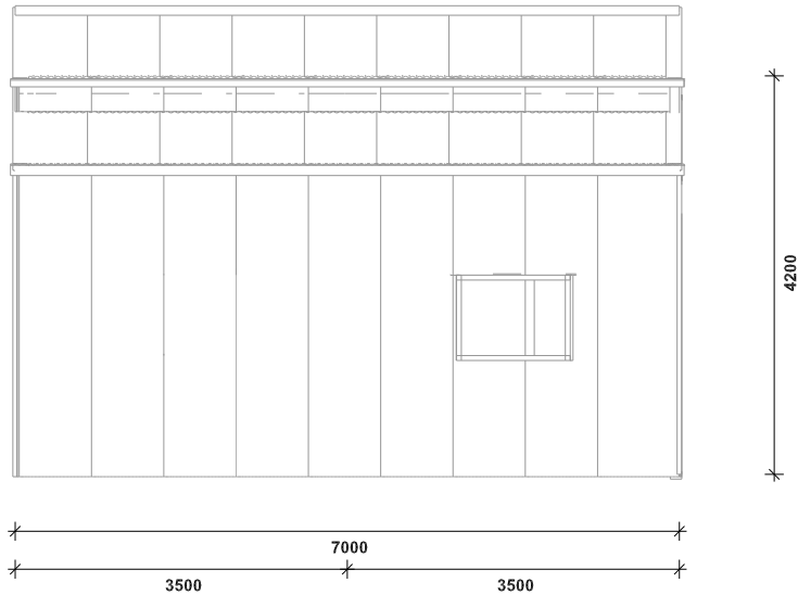
Elevation 1
