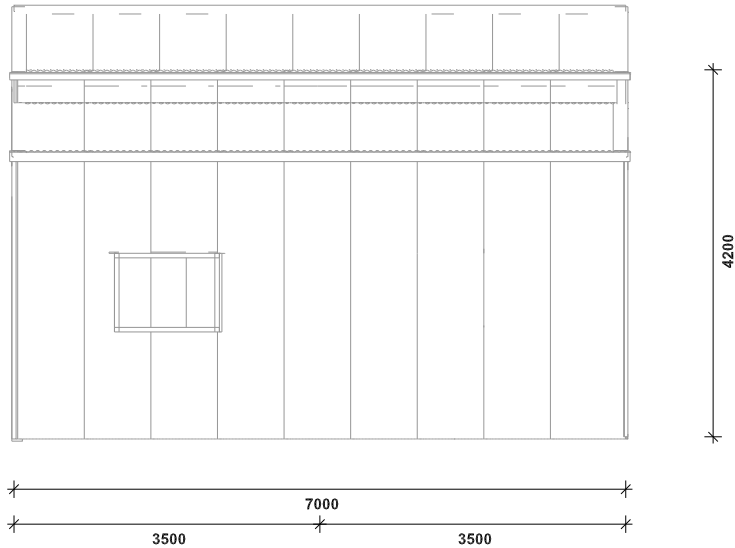
Elevation 3
