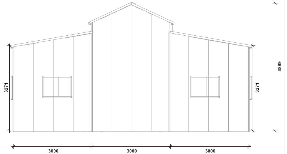
Elevation 2
