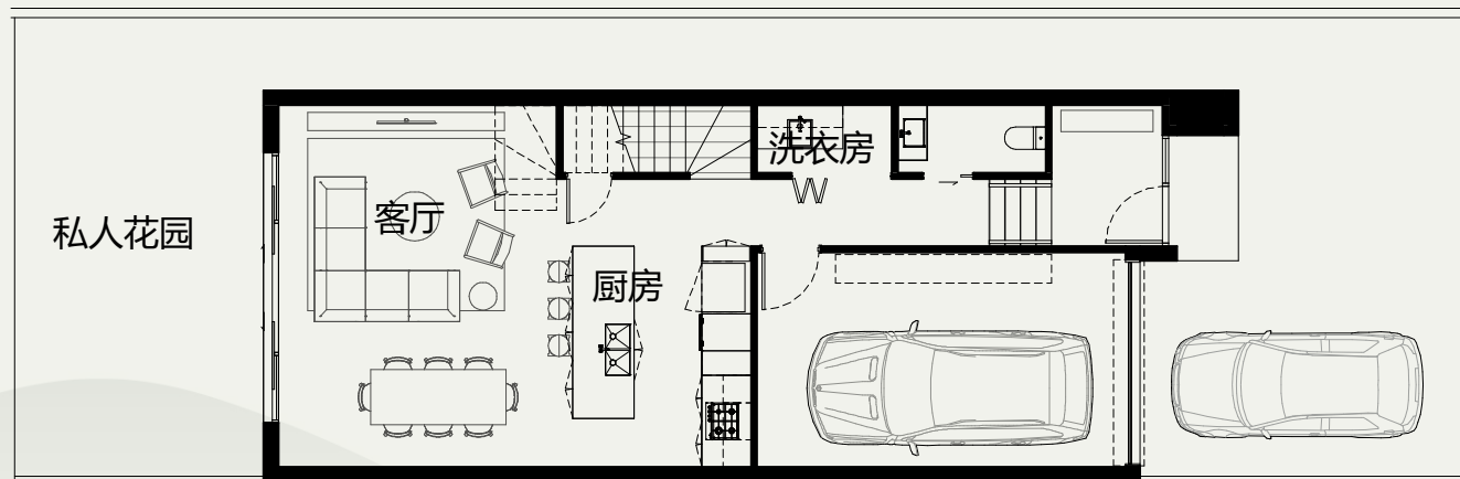
GROUND FLOOR 第一层
